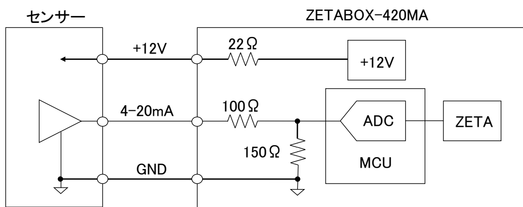
図 10 4-20mA インターフェース
