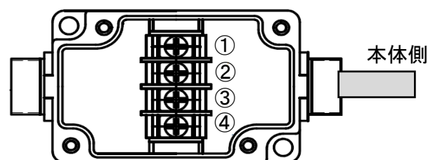
図 5 4-20mA 端子ボックス
