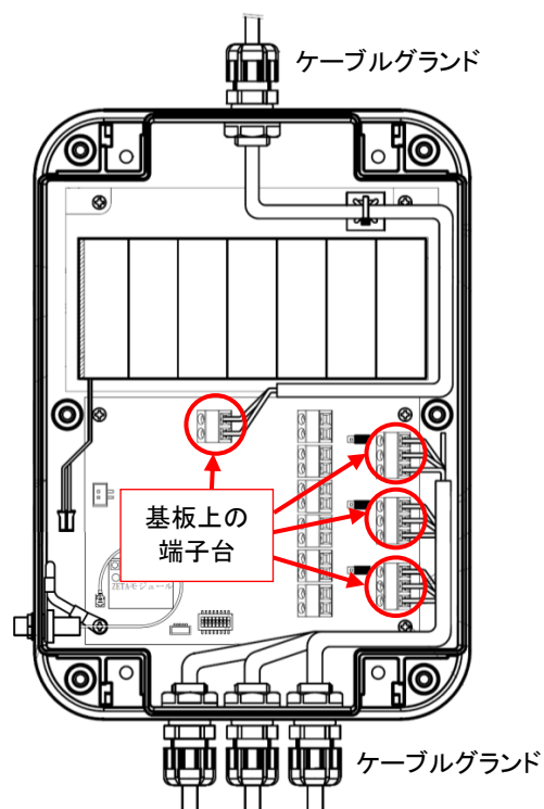
図 7 基板上的端子台位置
