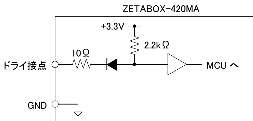
図 11 ドライ接点端子
