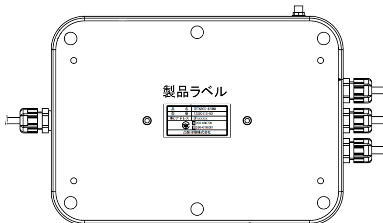
図 2 各部の名称
