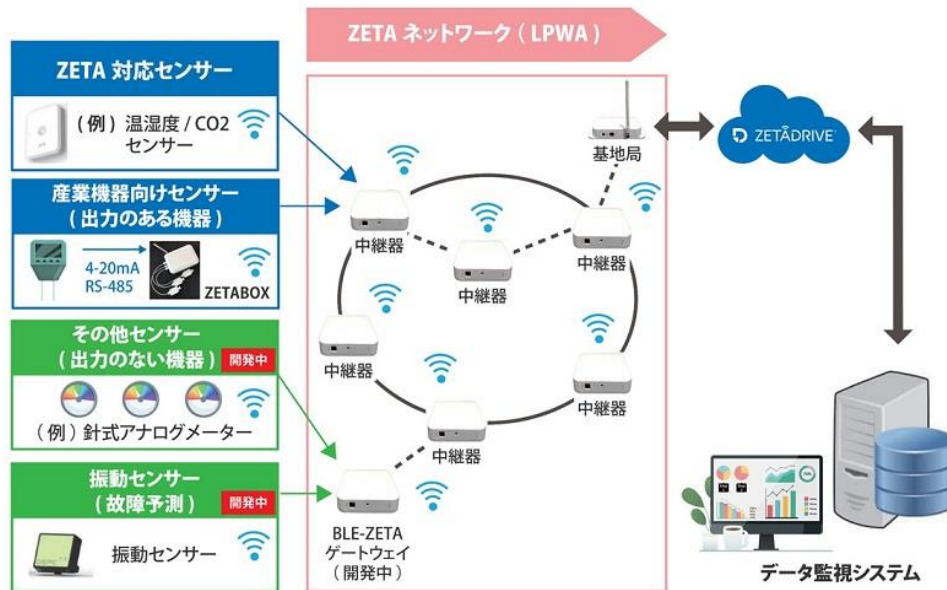
図 1 システム構成例
