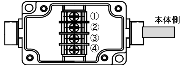
図 5 4-20mA 端子ボックス
