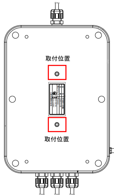
図 13 マウントブラケット取付位置
