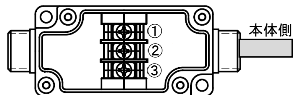
図 6 ドライ接点端子ボックス
