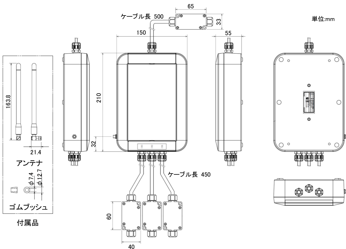
図3 外形寸法図
